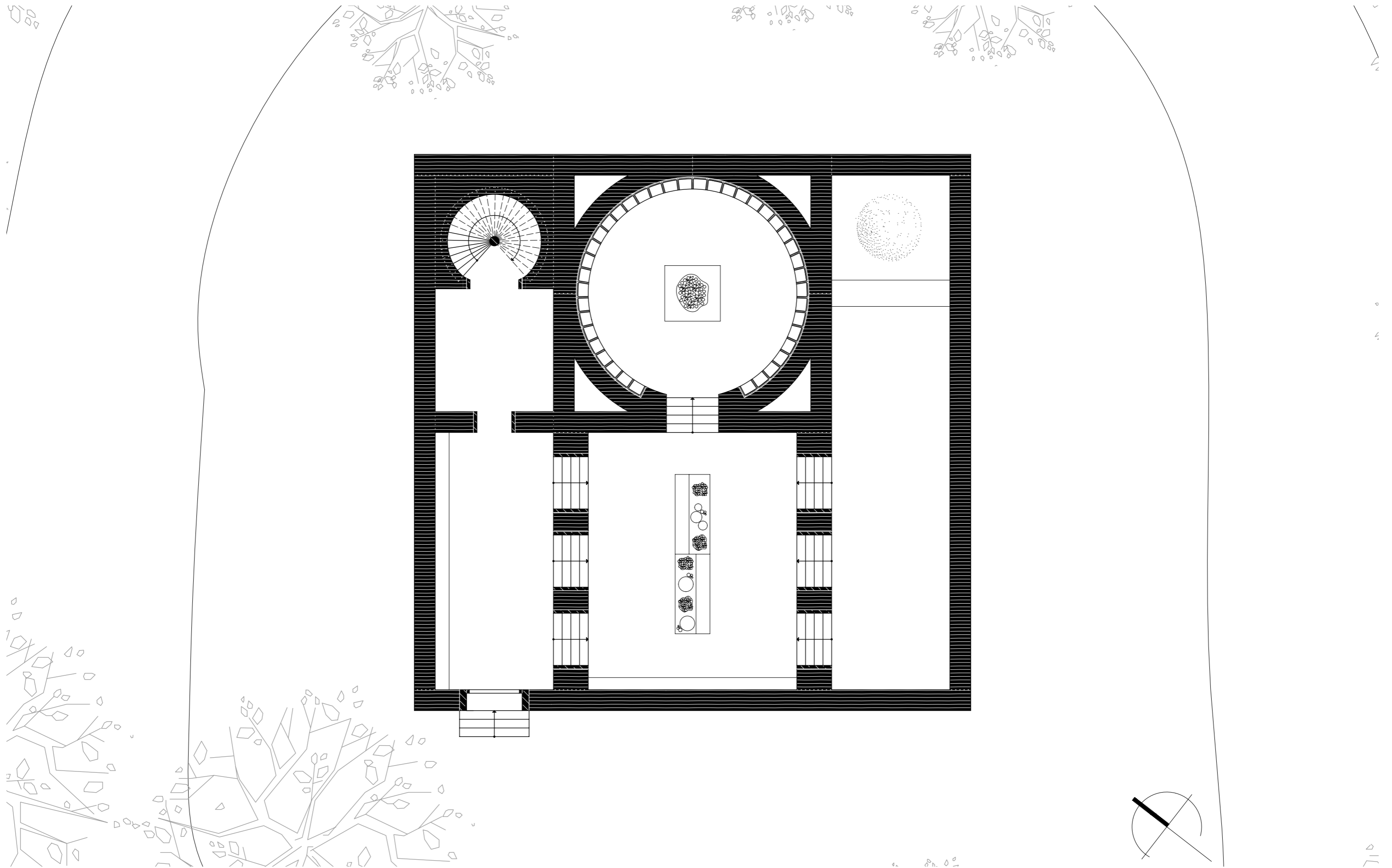
LEHMBAU GRUNDRISS ANTONIA LICHT
