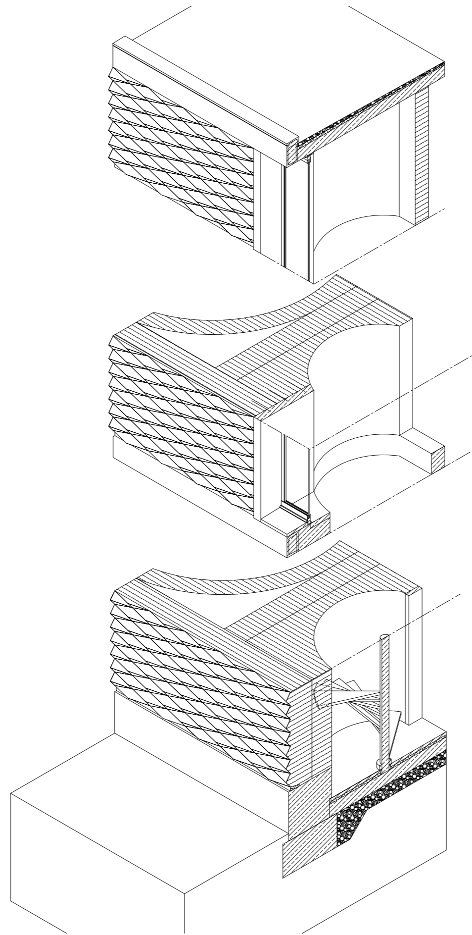
LEHMBAU FASSADENSCHNITT ANTONIA LICHT
