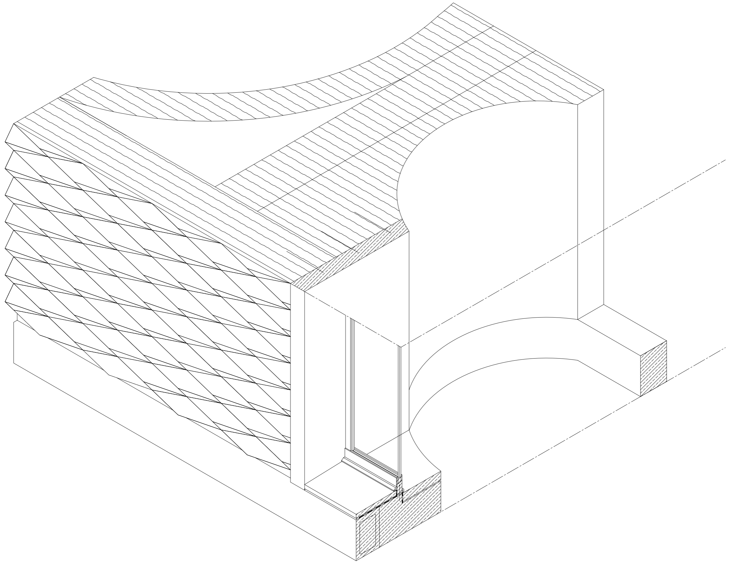
LEHMBAU DETAIL II ANTONIA LICHT
